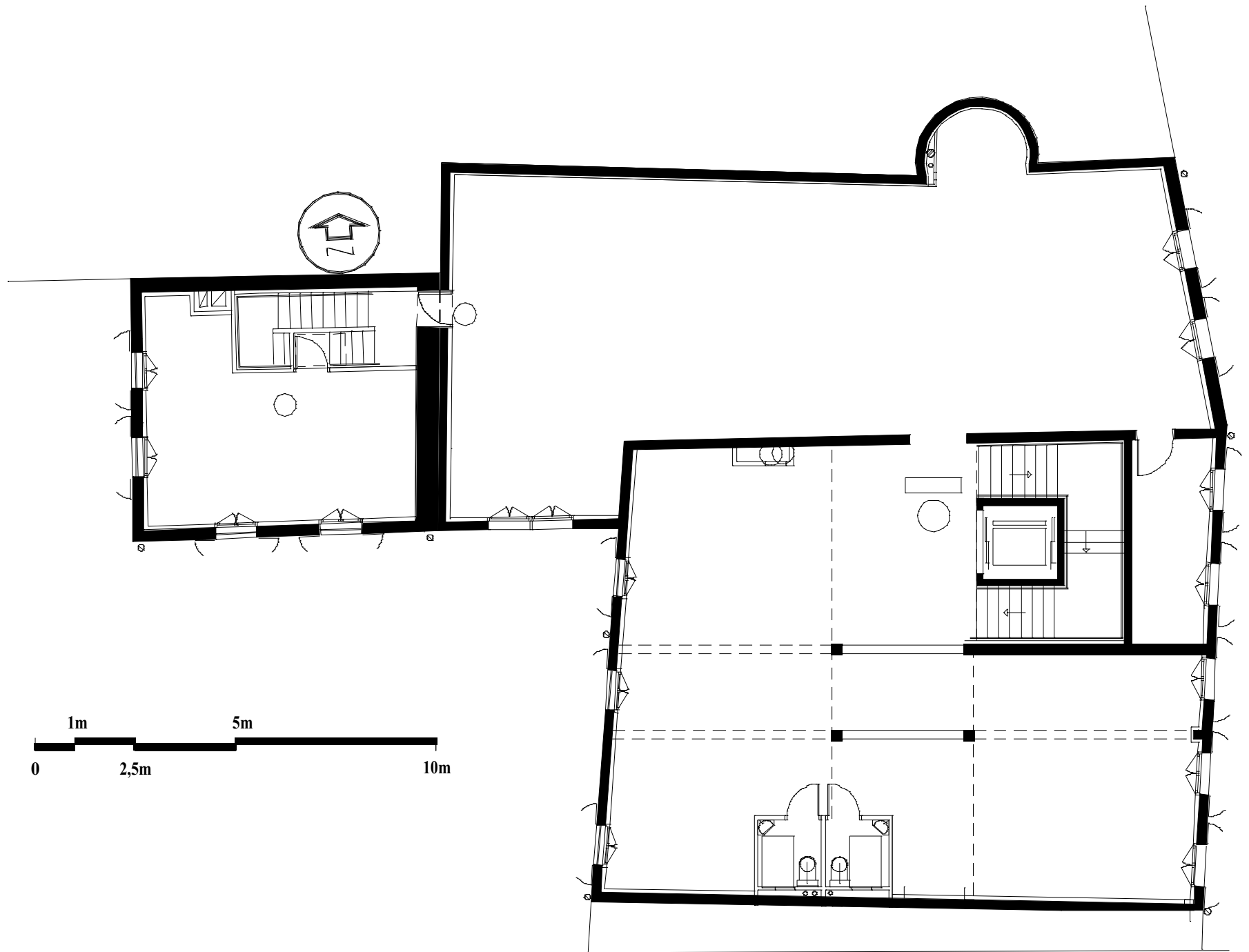
09C - Salle place du port (rue Fontenay): Plan 2ème Etage
